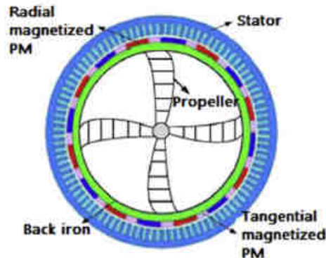
Figure 1 : Schéma de principe d'un propulseur Rim-Driven
