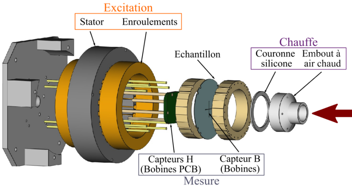
Figure 1: Système de caractérisation 2D avec système de mise en chauffe
