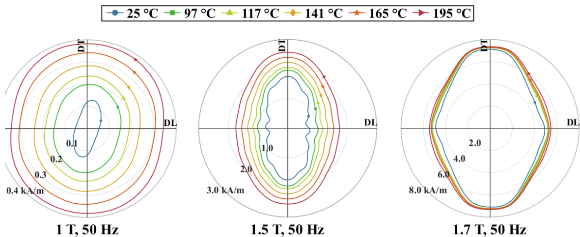
Figure 2: Vecteurs H représentés dans un plan 2D pour une induction de 1T(gauche), 1.5T(centre) et 1.7T(droite), 50Hz constante tournante pour différentes températures.
